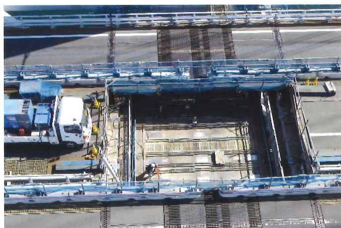
③(旧)大型伸縮装置撤去状況
