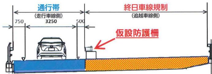
追越車線規制概略断面図
