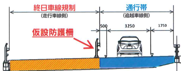
走行車線規制概略断面図
